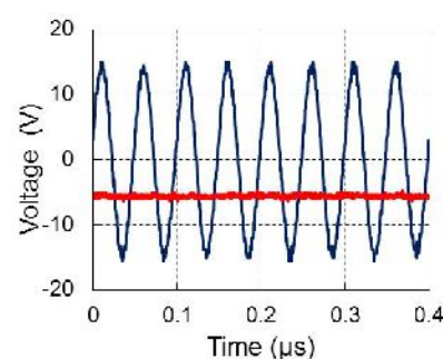
図 3 塗布結晶化法による有機整流回路による DC 出力
