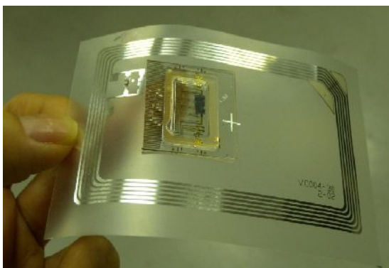
開発した電子タグ
