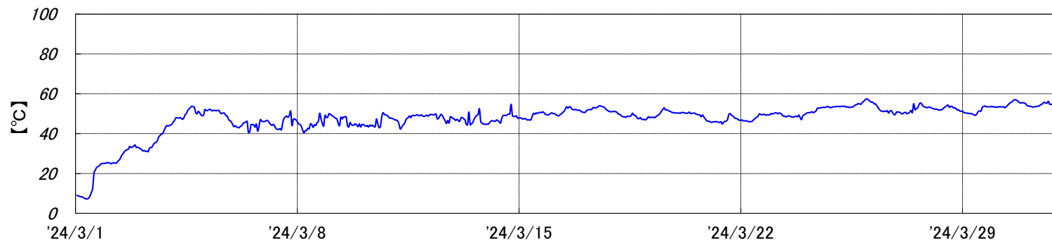
焼却炉 排ガス温度[2024年3月実績]
