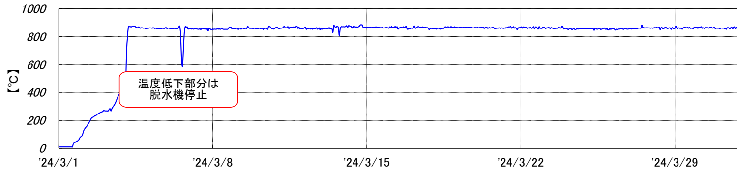
焼却炉 燃烧温度[2024年3月実績]
