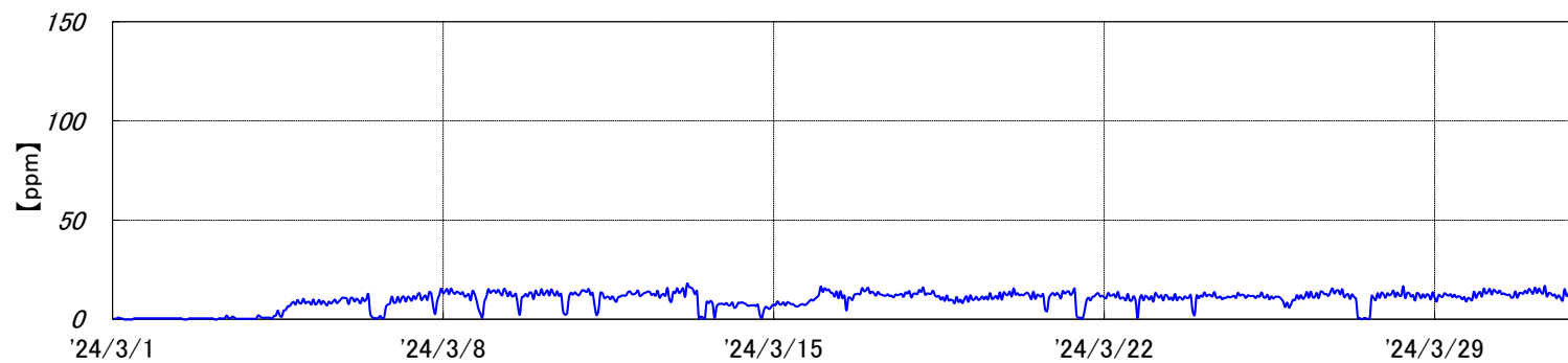
焼却炉 排ガスCO濃度[2024年3月実績]
