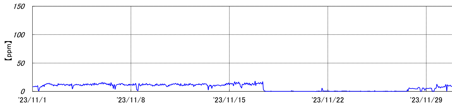
烧却炉 排ガスCO濃度[2023年11月実績]
