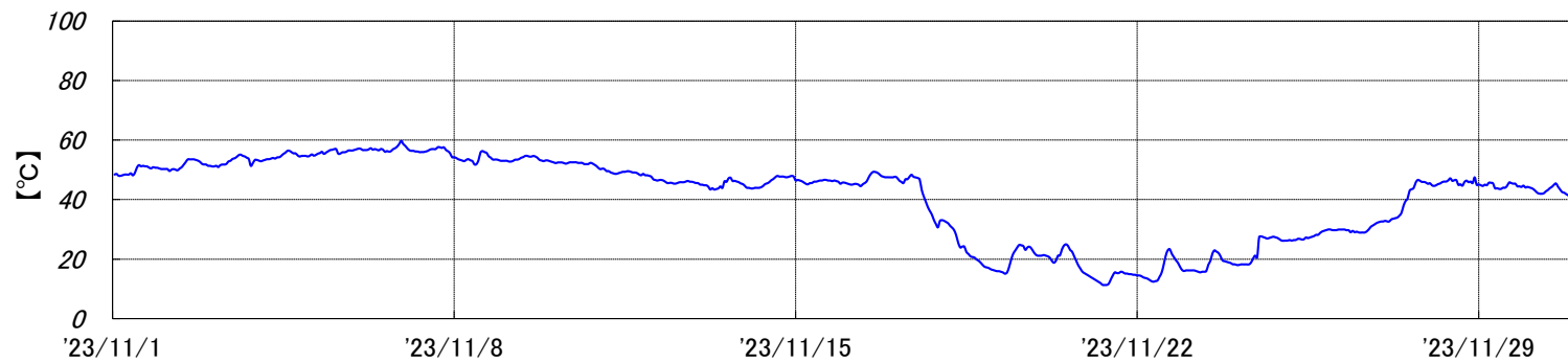
烧却炉 排ガス温度[2023年11月実績]
