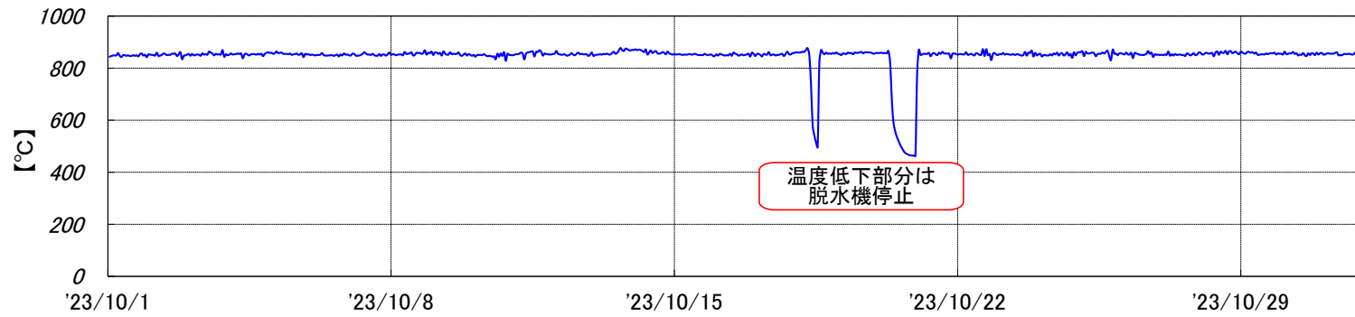
焼却炉 燃烧温度[2023年10月実績]
