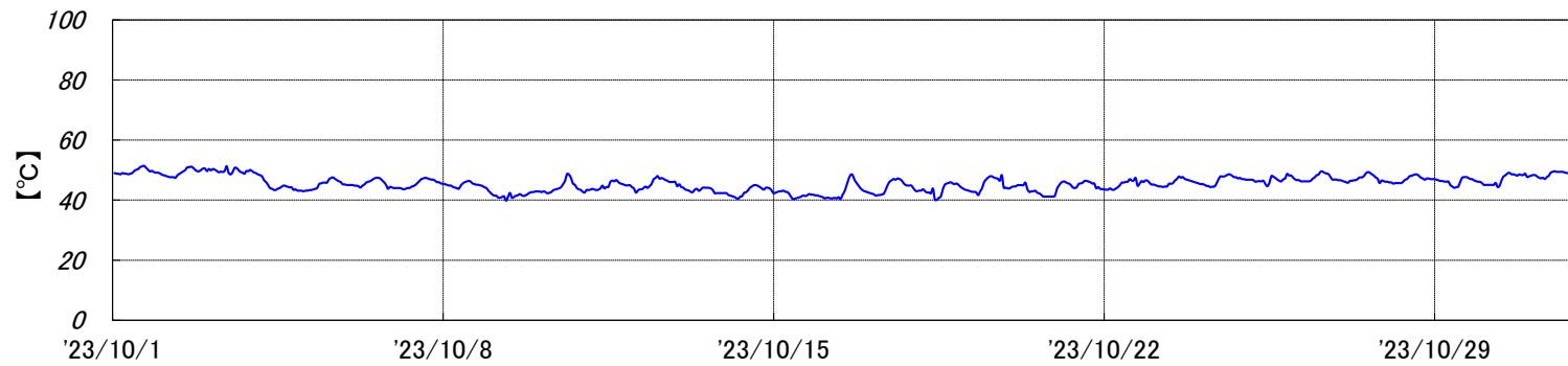
焼却炉 排ガス温度[2023年10月実績]
