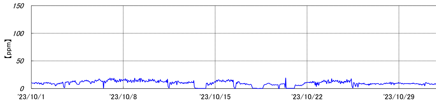
焼却炉 排ガスCO濃度[2023年10月実績]
