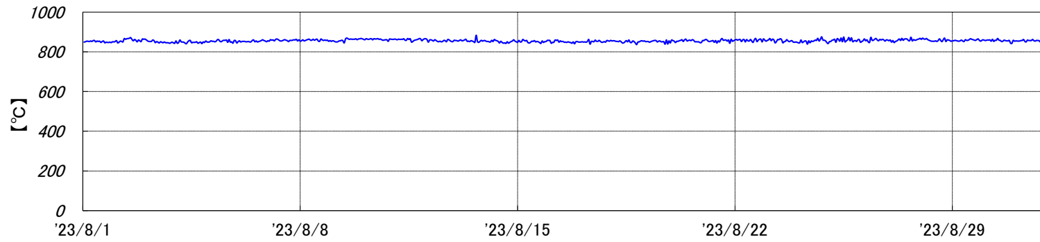
焼却炉 燃烧温度[2023年8月実績]
