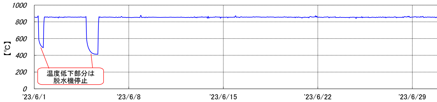
焼却炉 燃烧温度[2023年6月実績]
