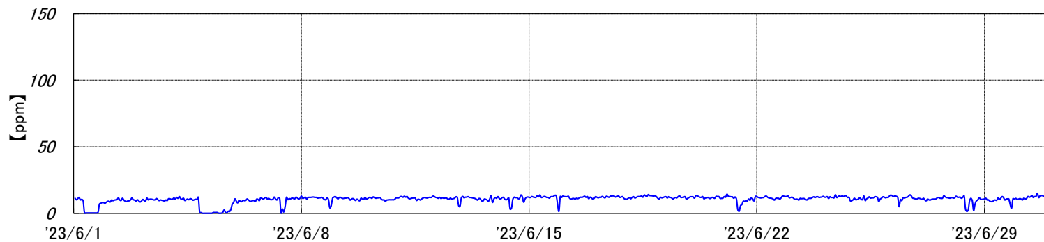
焼却炉 排ガスCO濃度[2023年6月実績]
