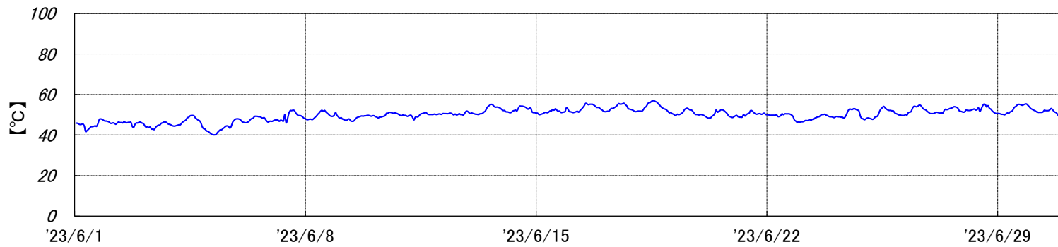
焼却炉 排ガス温度[2023年6月実績]
