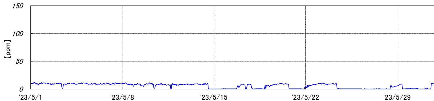
焼却炉 排ガスCO濃度[2023年5月実績]
