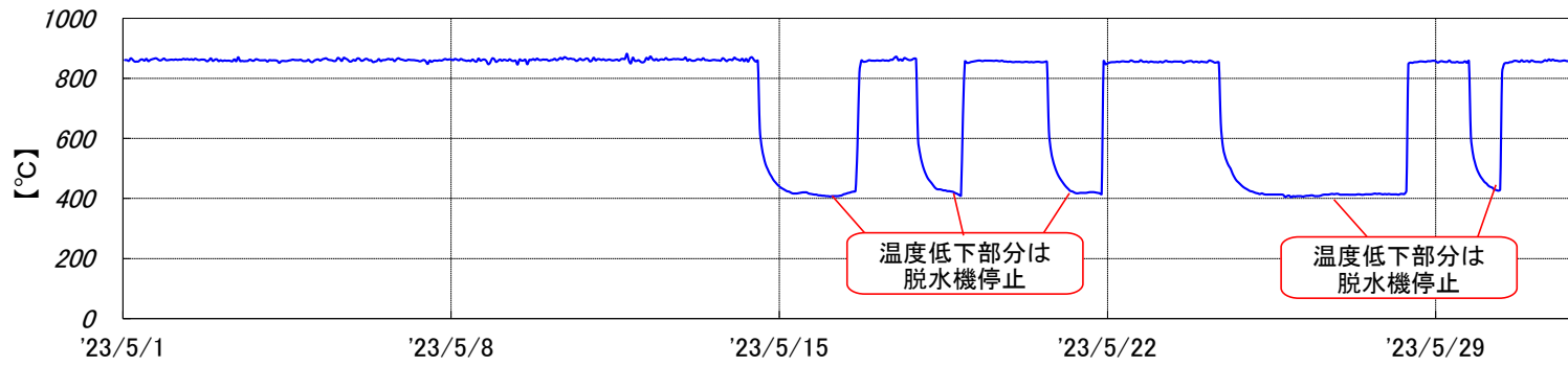
焼却炉 燃烧温度[2023年5月実績]
