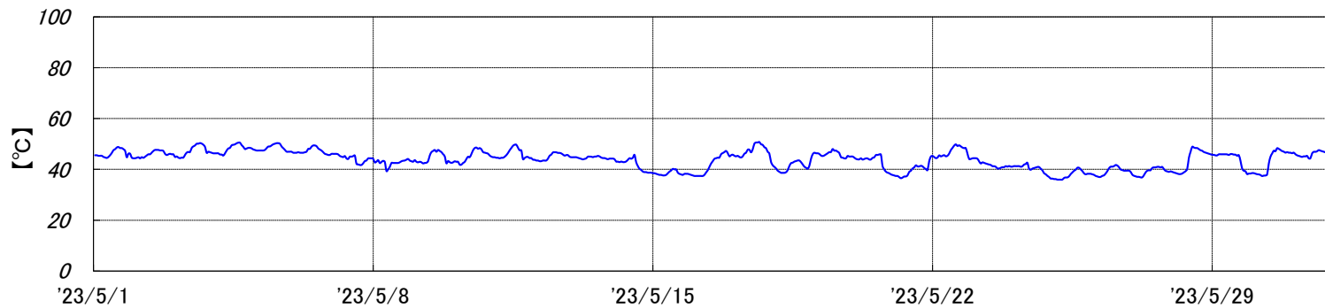
焼却炉 排ガス温度[2023年5月実績]
