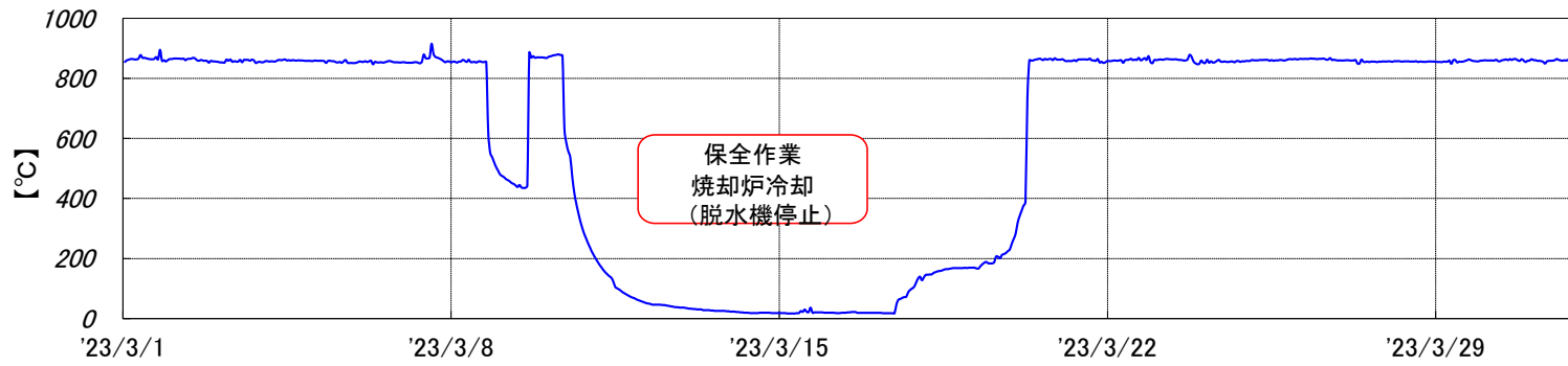
焼却炉 燃烧温度[2023年3月実績]
