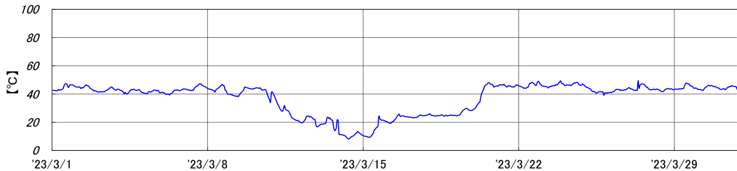
焼却炉 排ガス温度[2023年3月実績]
