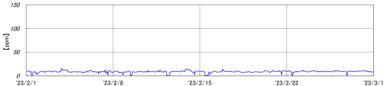
烧却炉 排ガスCO濃度[2023年2月実績]
