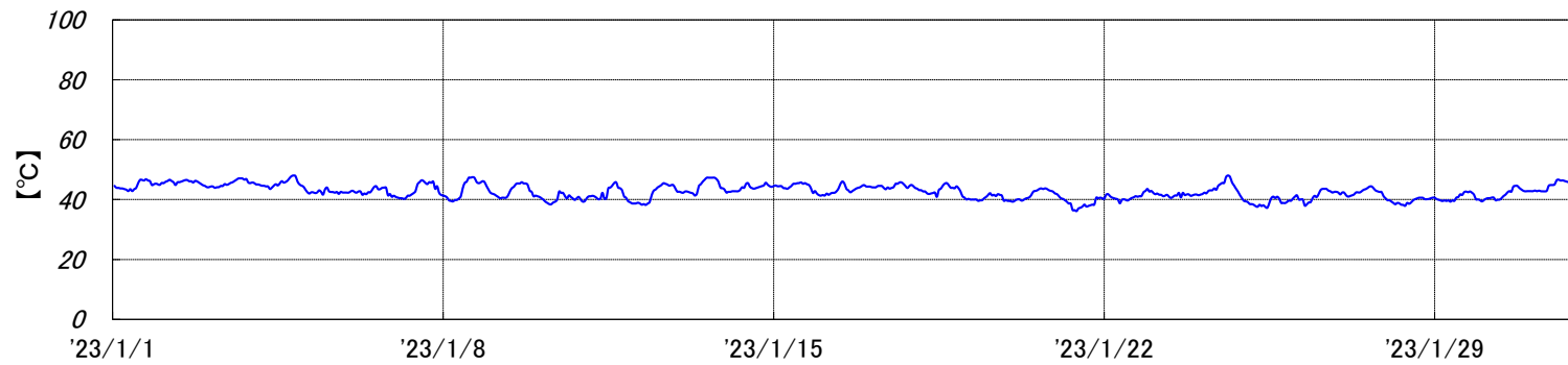
焼却炉 排ガス温度[2023年1月実績]
