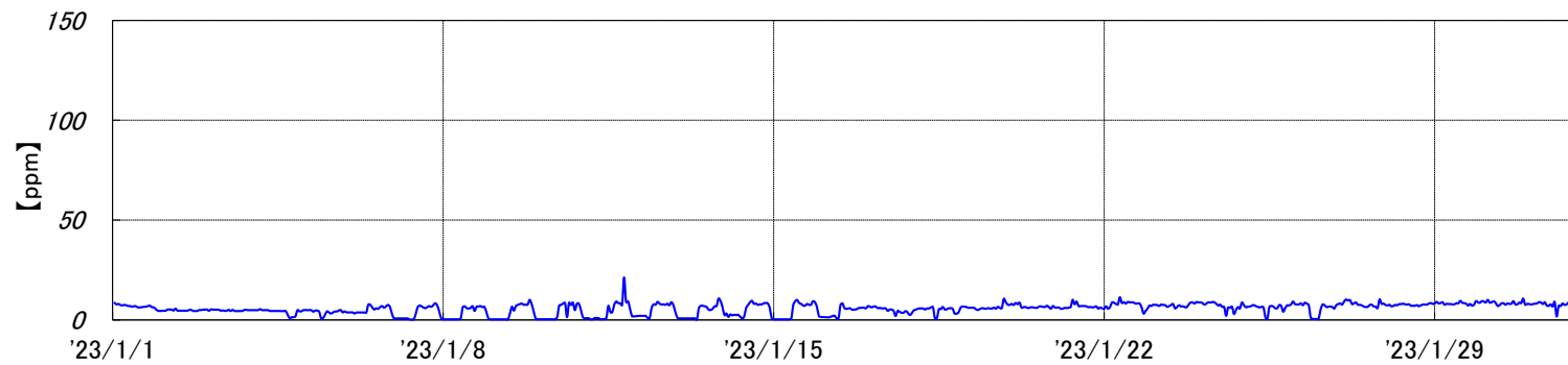
焼却炉 排ガスCO濃度[2023年1月実績]
