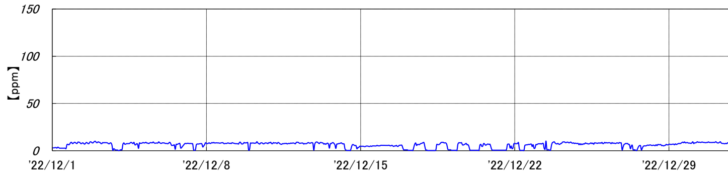
烧却炉 排ガスCO濃度[2022年12月実績]
