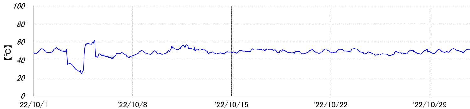
焼却炉 排ガス温度[2022年10月実績]
