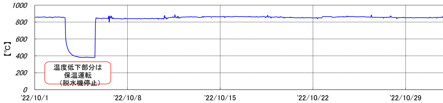
焼却炉 燃烧温度[2022年10月実績]
