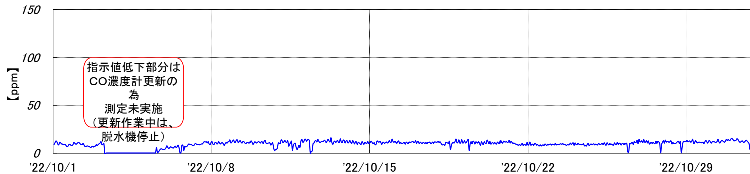
焼却炉 排ガスCO濃度[2022年10月実績]
