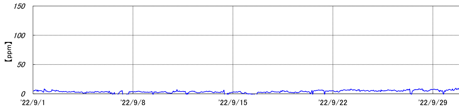
焼却炉 排ガスCO濃度[2022年9月実績]
