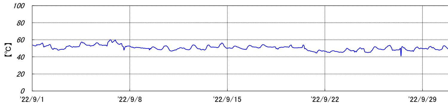
焼却炉 排ガス温度[2022年9月実績]
