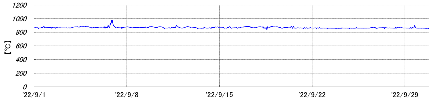
焼却炉 燃烧温度[2022年9月実績]
