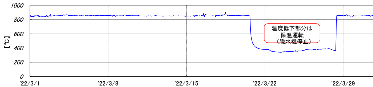
烧却炉 燃烧温度[2022年3月実績]
