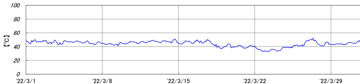
烧却炉 排ガス温度[2022年3月実績]
