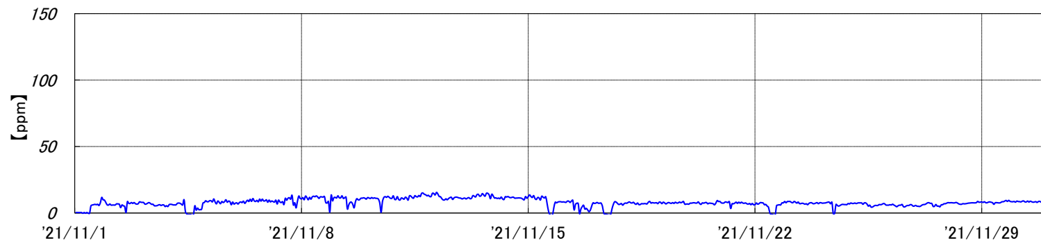
烧却炉 排ガスCO濃度[2021年11月実績]
