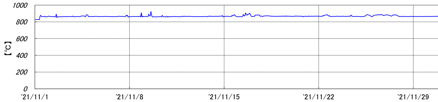
烧却炉 燃烧温度[2021年11月実績]
