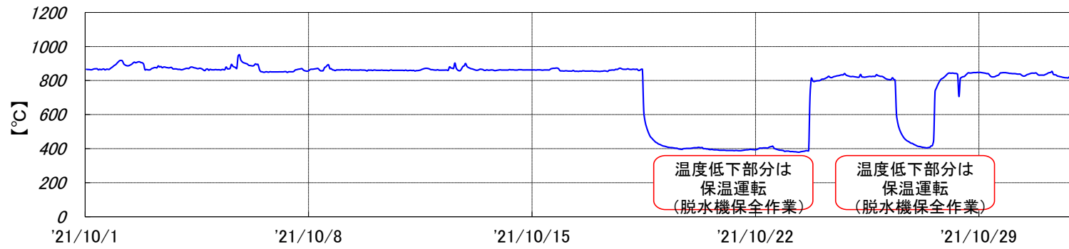
焼却炉 燃烧温度[2021年10月実績]
