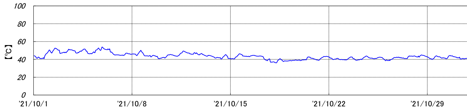
焼却炉 排ガス温度[2021年10月実績]
