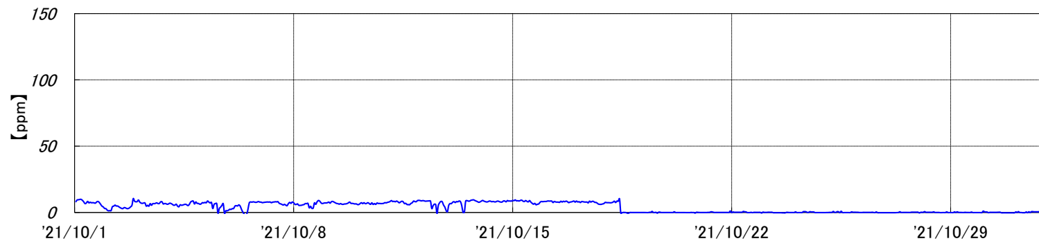
焼却炉 排ガスCO濃度[2021年10月実績]
