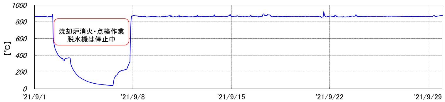
焼却炉 燃烧温度[2021年9月実績]
