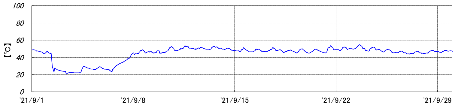
焼却炉 排ガス温度[2021年9月実績]
