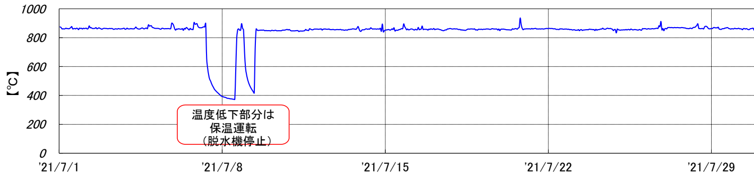
烧却炉 燃烧温度[2021年7月実績]
