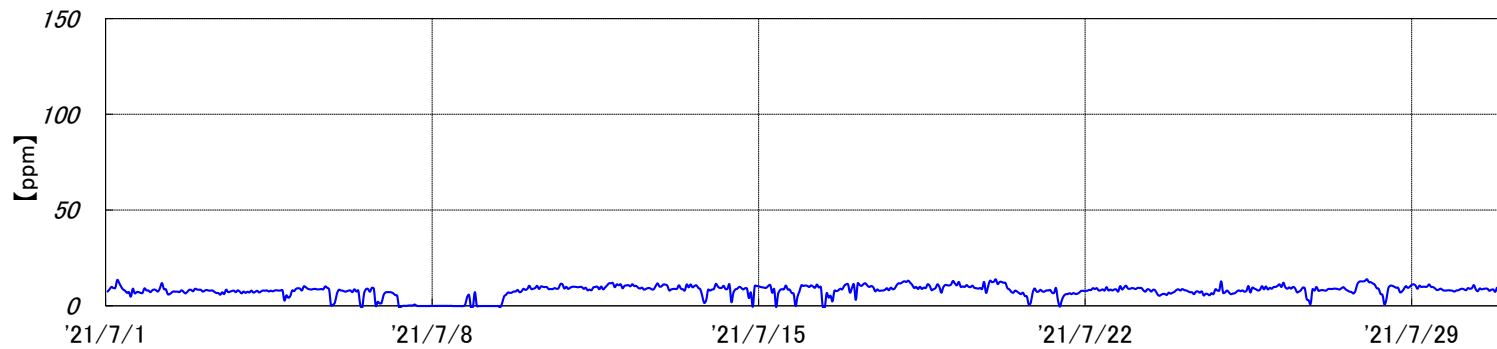
烧却炉 排ガスCO濃度[2021年7月実績]
