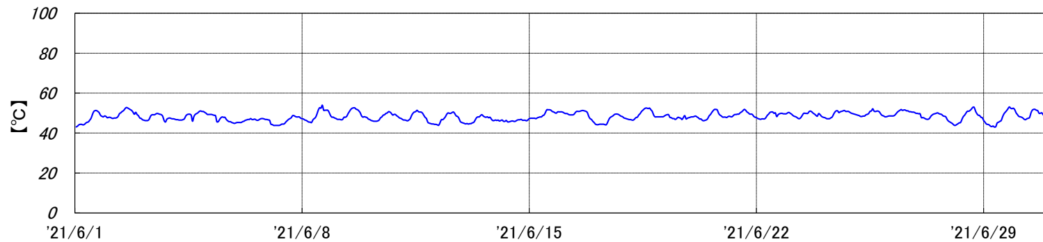
烧却炉 排ガス温度[2021年6月実績]
