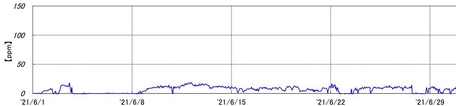
烧却炉 排ガスCO濃度[2021年6月実績]
