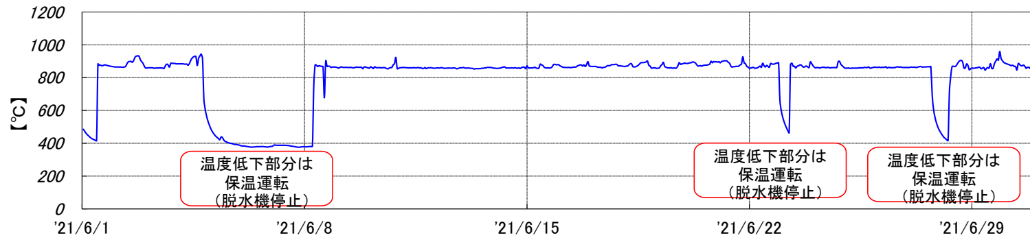
烧却炉 燃烧温度[2021年6月実績]
