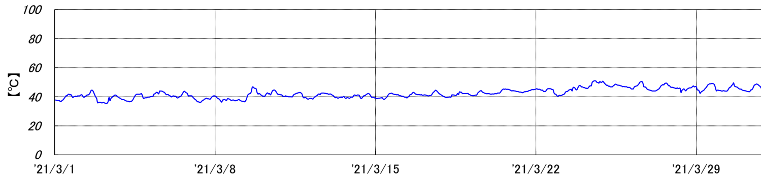
焼却炉 排ガス温度[2021年3月実績]
