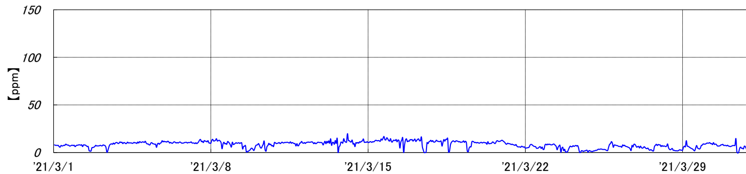
焼却炉 排ガスCO濃度[2021年3月実績]
