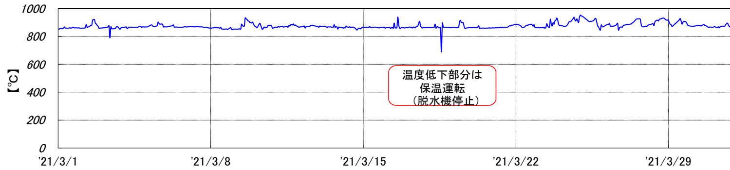
焼却炉 燃烧温度[2021年3月実績]
