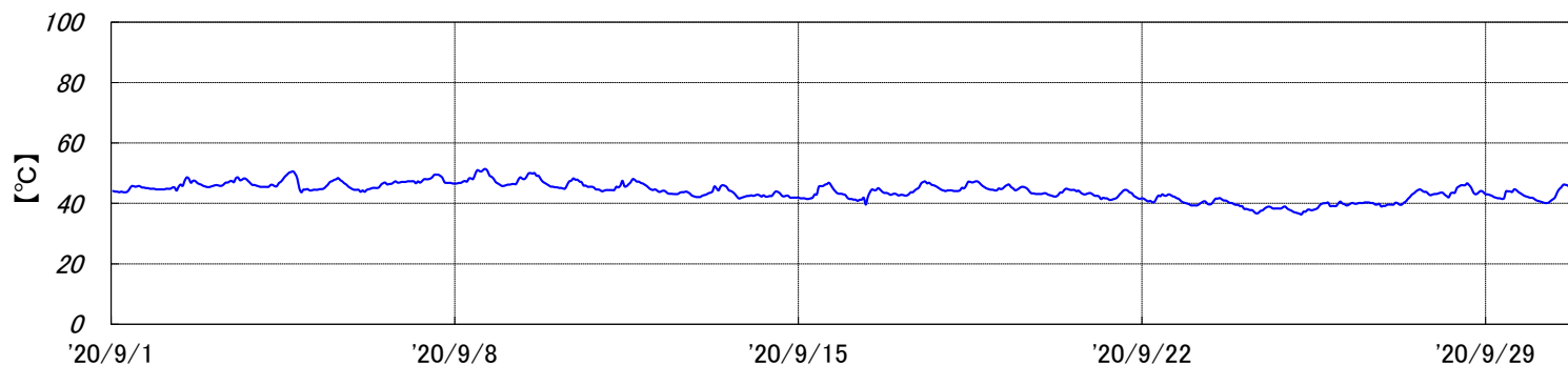
焼却炉 排ガス温度[2020年9月実績]
