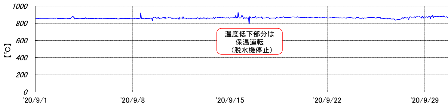
焼却炉 燃烧温度[2020年9月実績]
