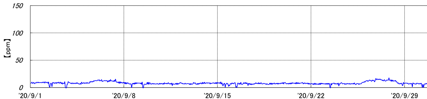
焼却炉 排ガスCO濃度[2020年9月実績]
