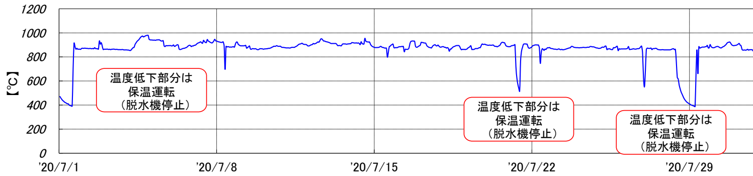
焼却炉 燃烧温度[2020年7月実績]
