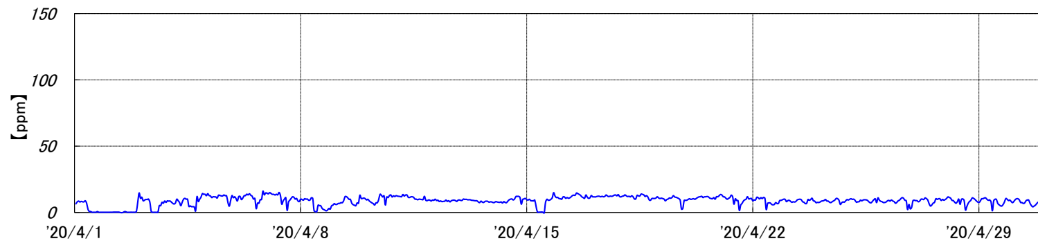
焼却炉 排ガスCO濃度[2020年4月実績]
