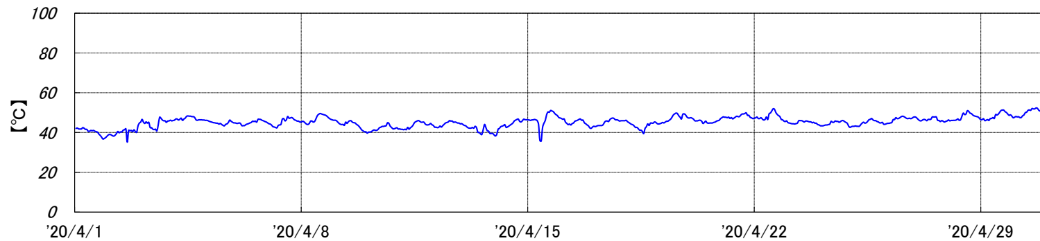
焼却炉 排ガス温度[2020年4月実績]
