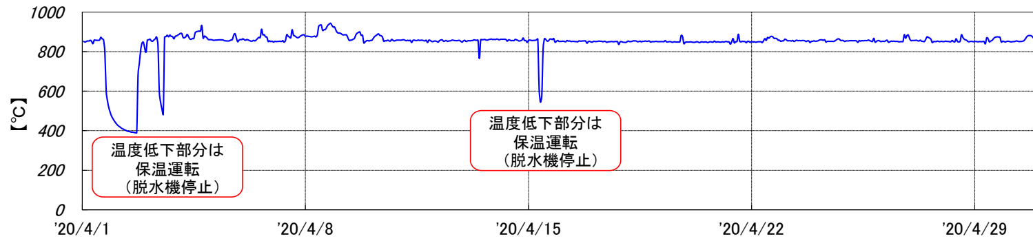
焼却炉 燃烧温度[2020年4月実績]
