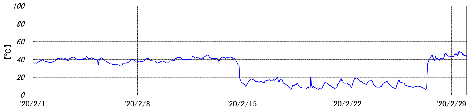
烧却炉 排ガス温度[2020年2月実績]
