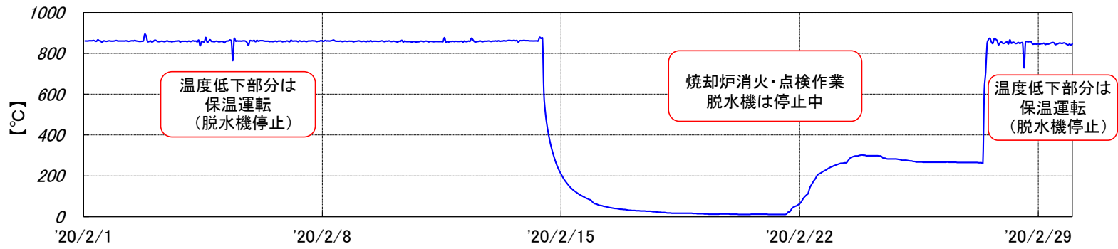
烧却炉 燃烧温度[2020年2月実績]
