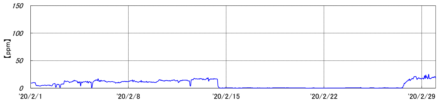
烧却炉 排ガスCO濃度[2020年2月実績]
