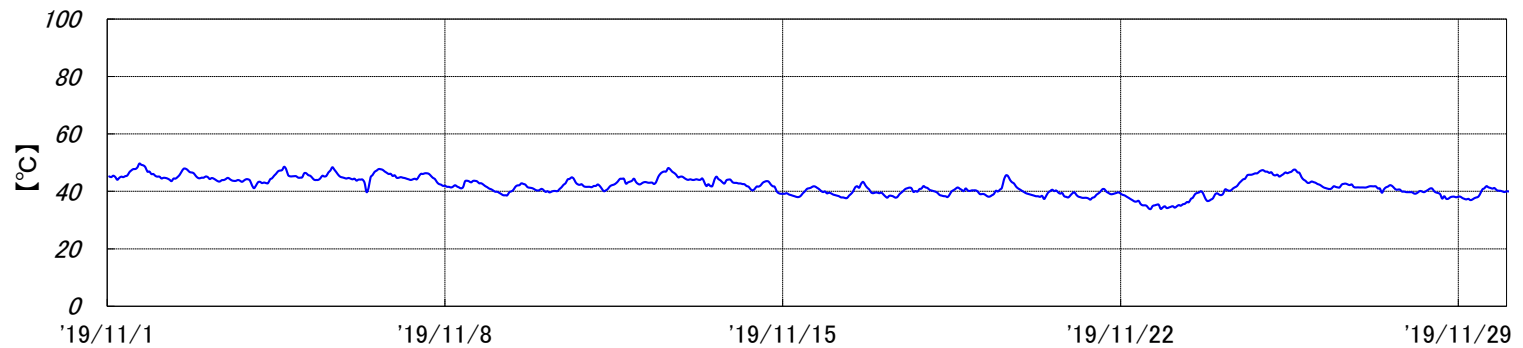
烧却炉 排ガス温度[2019年11月実績]
