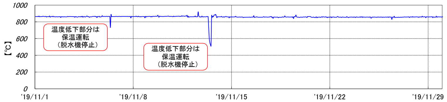
烧却炉 燃烧温度[2019年11月実績]
