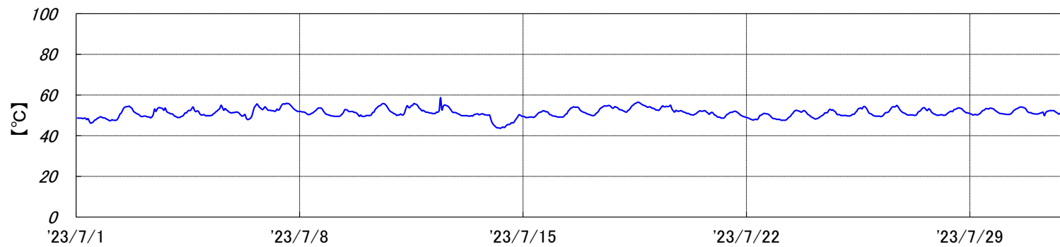
焼却炉 排ガス温度[2023年7月実績]
