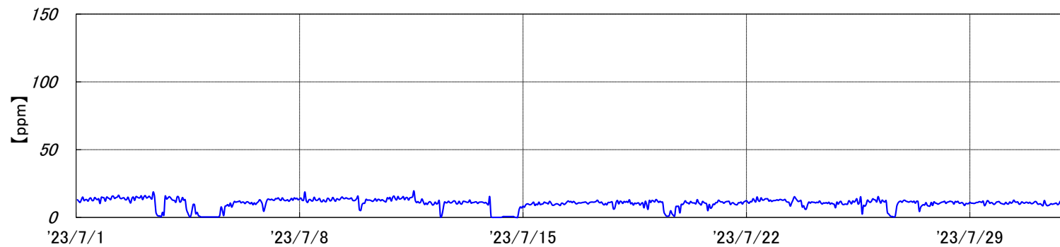
焼却炉 排ガスCO濃度[2023年7月実績]
