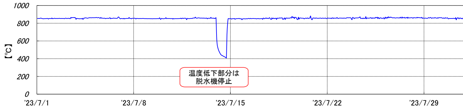
焼却炉 燃烧温度[2023年7月実績]
