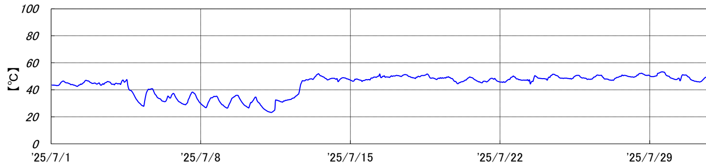
焼却炉 排ガス温度〔2025年7月実績〕
