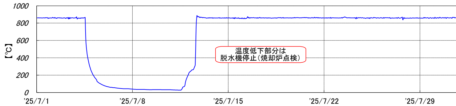
焼却炉 燃烧温度〔2025年7月実績〕
