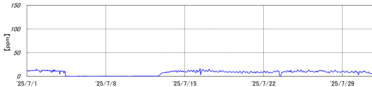
焼却炉 排ガスCO濃度〔2025年7月実績〕
