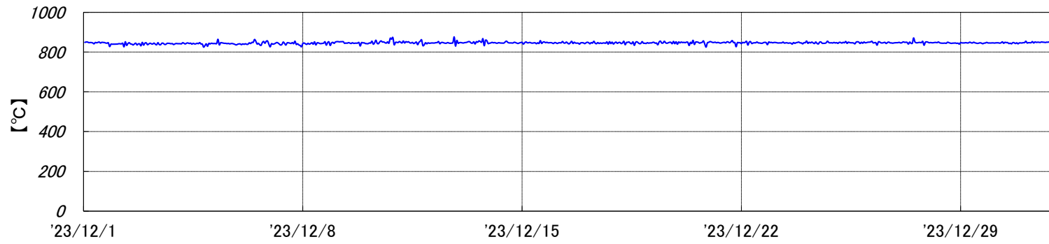
烧却炉 燃烧温度[2023年12月実績]
