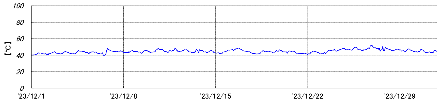
烧却炉 排ガス温度[2023年12月実績]
