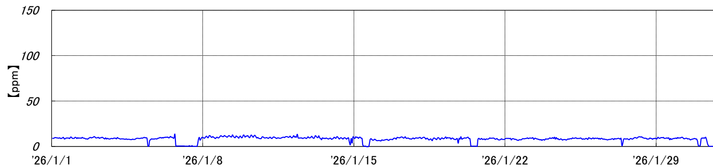
焼却炉 排ガスCO濃度〔2026年1月実績〕
