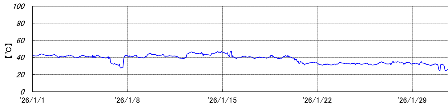
焼却炉 排ガス温度〔2026年1月実績〕
