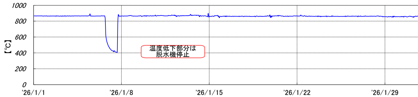
焼却炉 燃烧温度〔2026年1月実績〕
