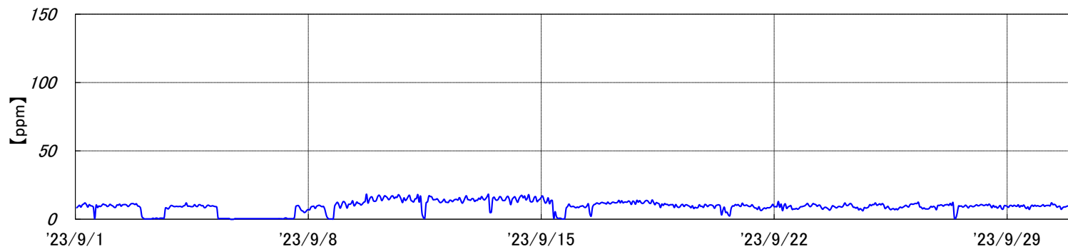
焼却炉 排ガスCO濃度[2023年9月実績]
