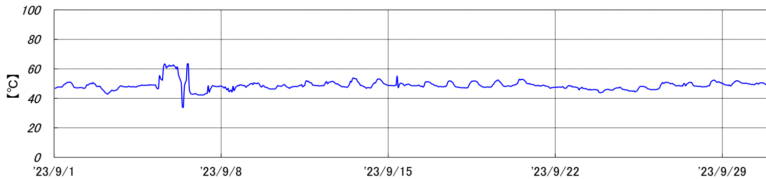
焼却炉 排ガス温度[2023年9月実績]
