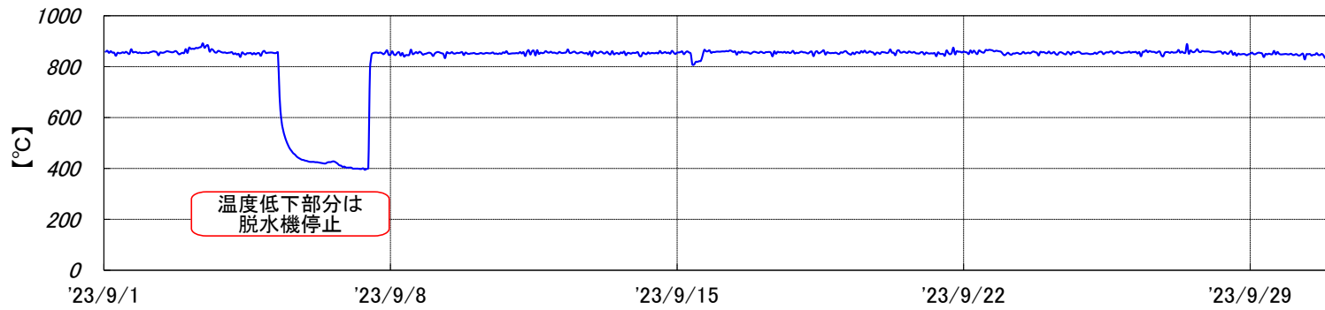
焼却炉 燃烧温度[2023年9月実績]
