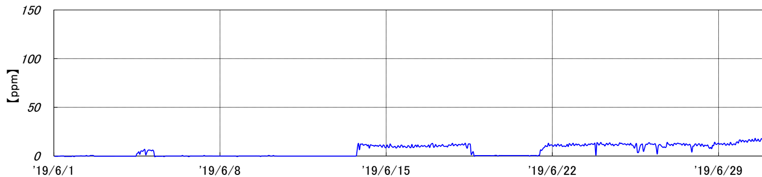
烧却炉 排ガスCO濃度[2019年6月実績]
