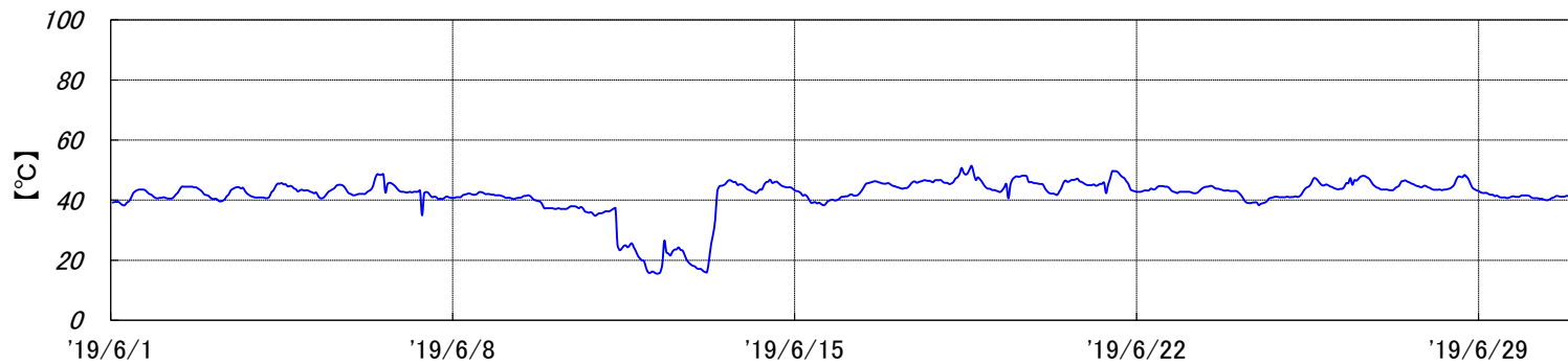
烧却炉 排ガス温度[2019年6月実績]
