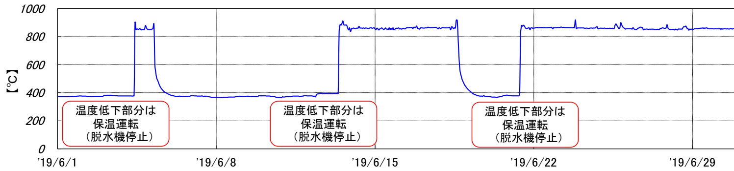
烧却炉 燃烧温度[2019年6月実績]
