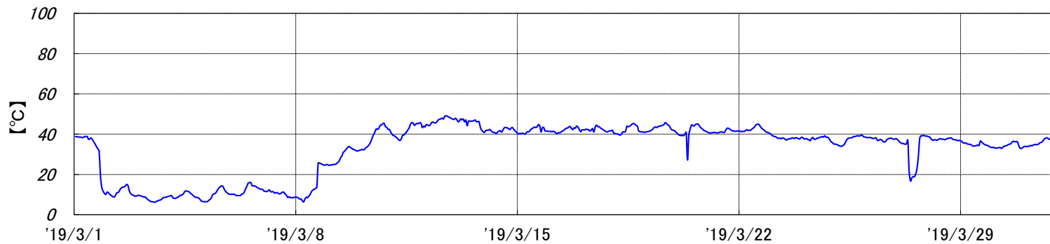
焼却炉 排ガス温度[2019年3月実績]
