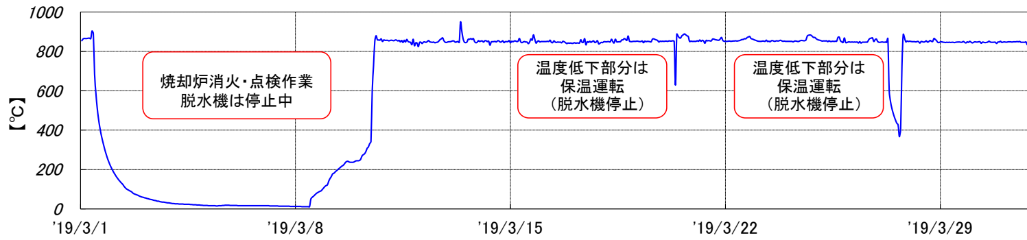
焼却炉 燃烧温度[2019年3月実績]
