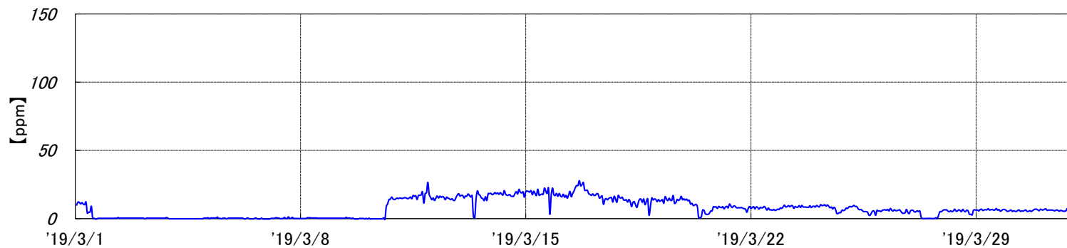
焼却炉 排ガスCO濃度[2019年3月実績]
