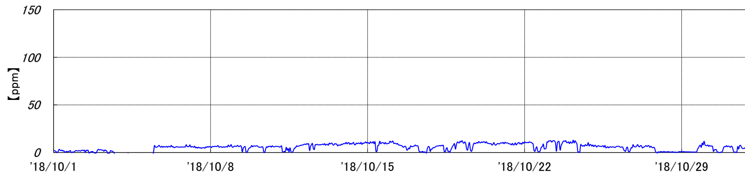
烧却炉 排ガスCO濃度[2018年10月実績]
