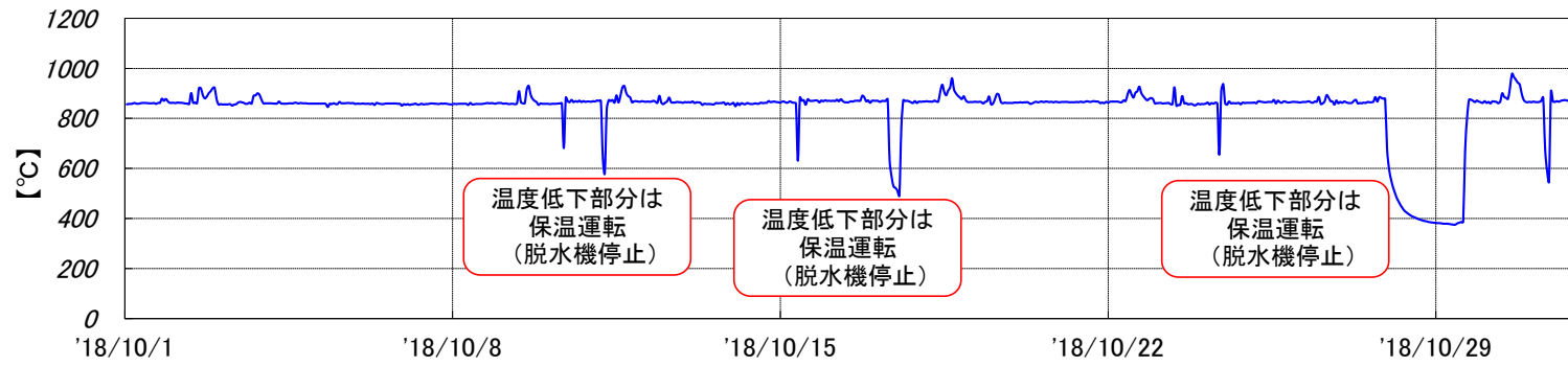
烧却炉 燃烧温度[2018年10月実績]
