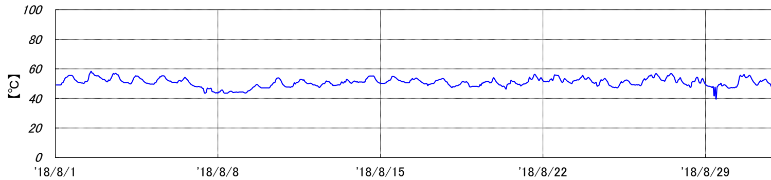
烧却炉 排ガス温度[2018年8月実績]
