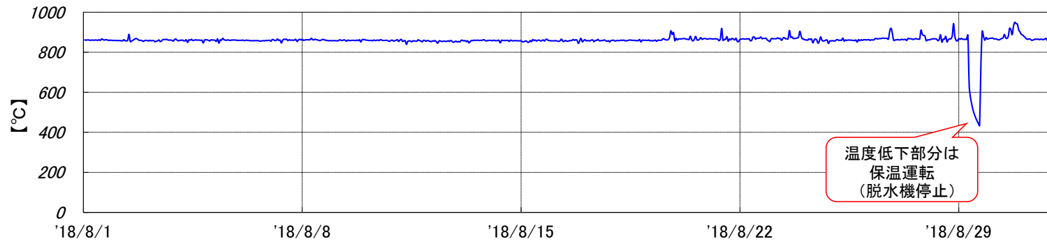
烧却炉 燃烧温度[2018年8月実績]
