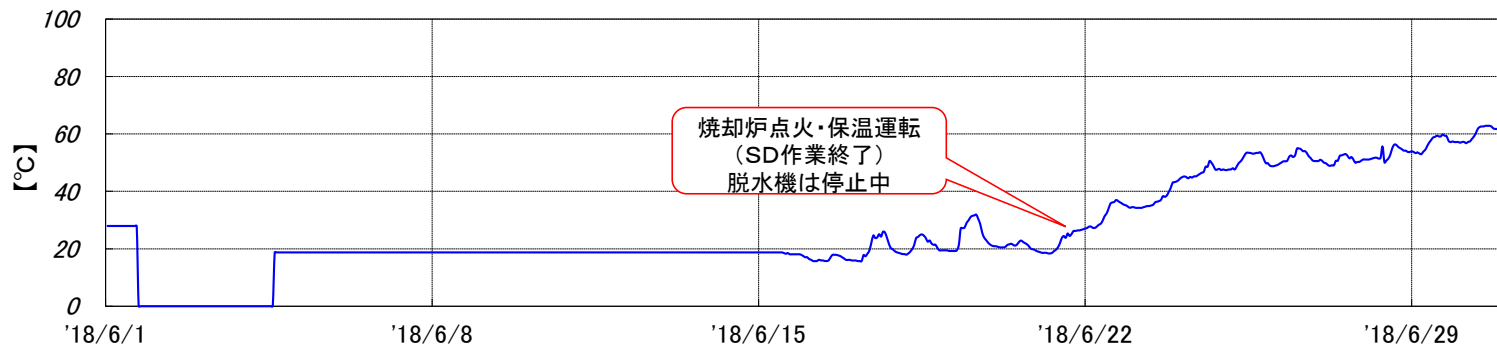
烧却炉 排ガス温度[2018年6月実績]
