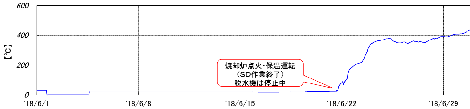
烧却炉 燃烧温度[2018年6月実績]
