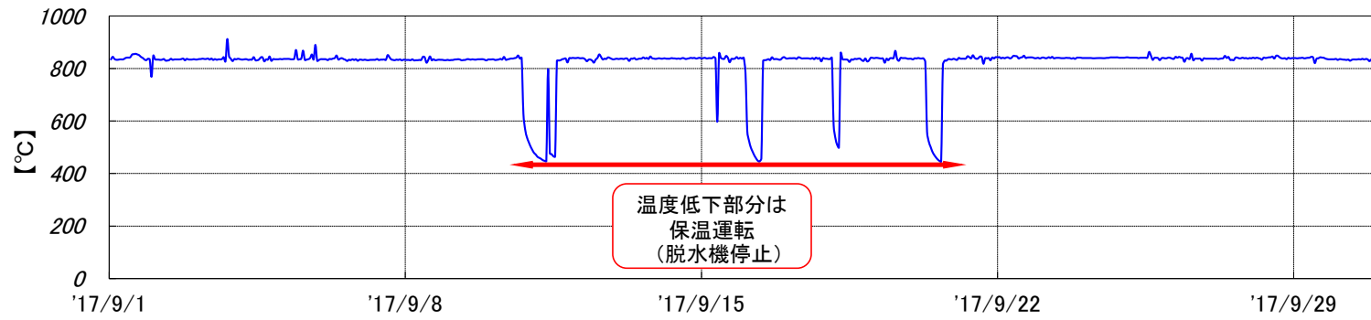
烧却炉 燃烧温度[2017年9月実績]
