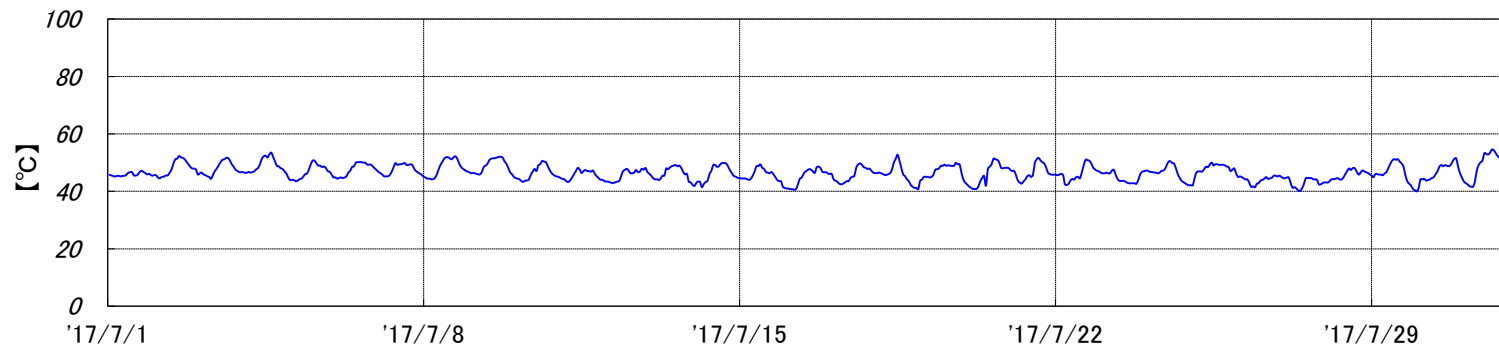
焼却炉 排ガス温度[2017年7月実績]
