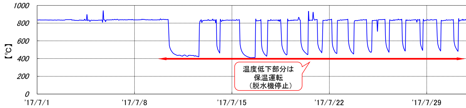
焼却炉 燃烧温度[2017年7月実績]
