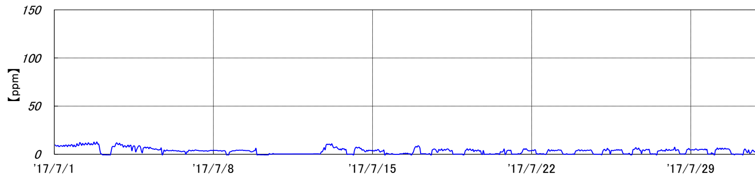
焼却炉 排ガスCO濃度[2017年7月実績]
