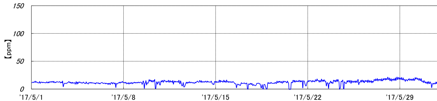
烧却炉 排ガスCO濃度[2017年5月実績]
