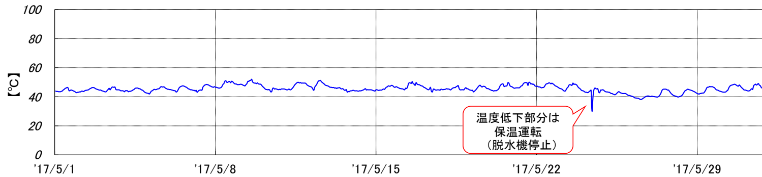
烧却炉 排ガス温度[2017年5月実績]
