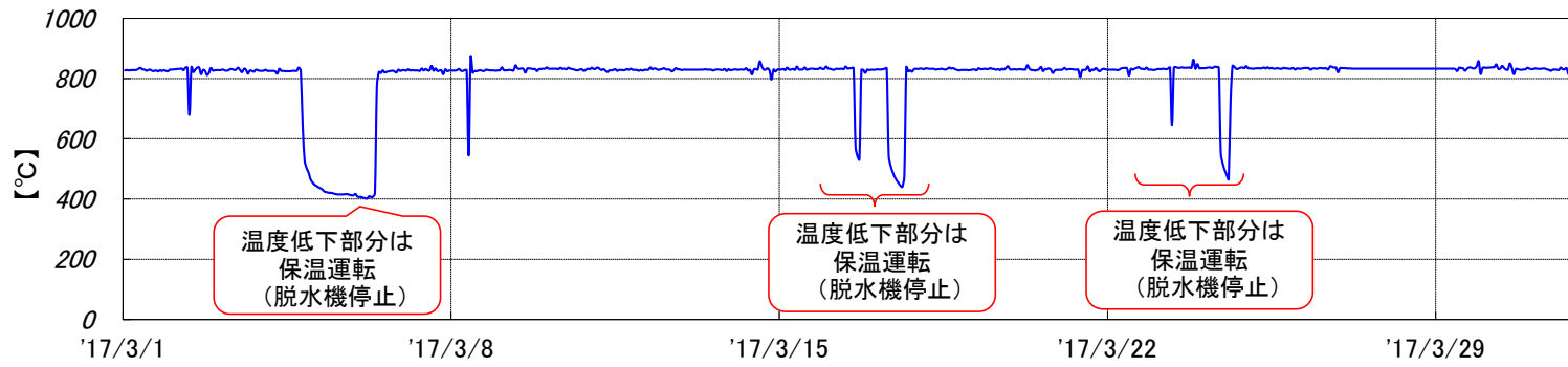
焼却炉 燃烧温度[2017年3月実績]
