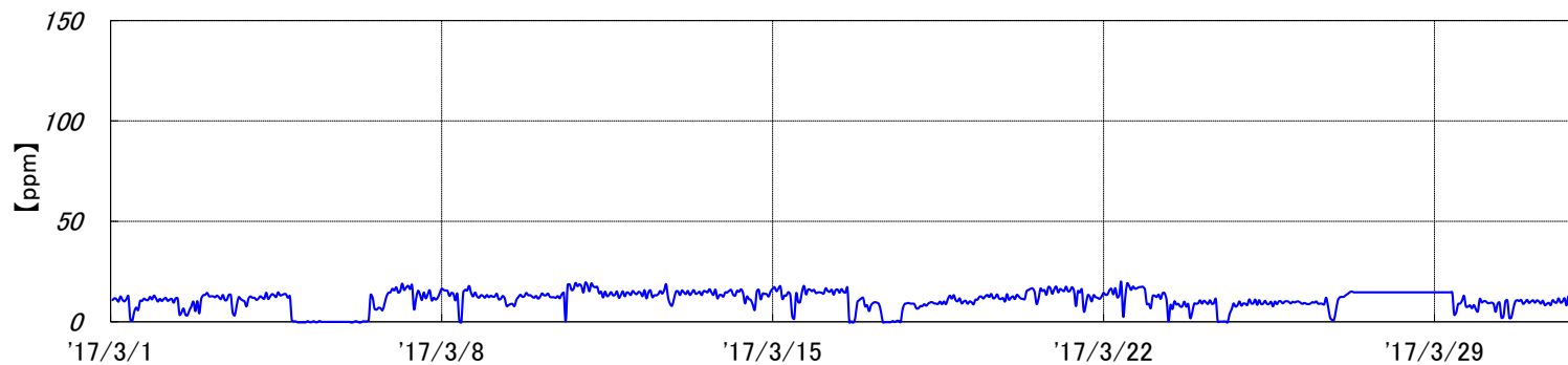
焼却炉 排ガスCO濃度[2017年3月実績]
