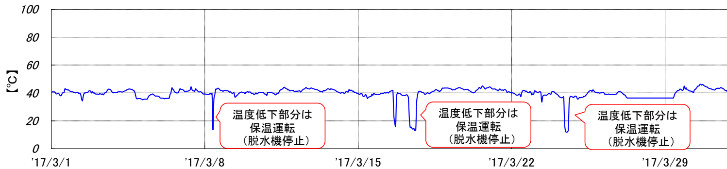
焼却炉 排ガス温度[2017年3月実績]
