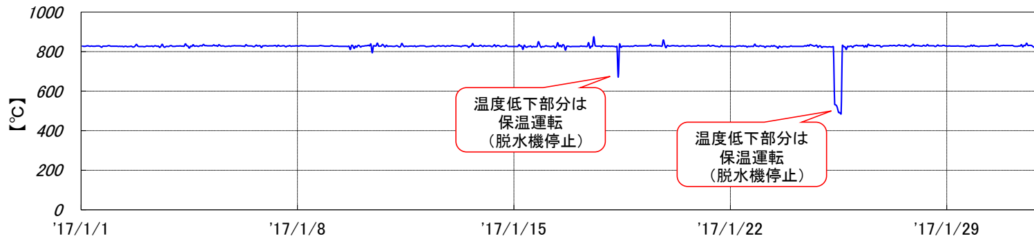
烧却炉 燃烧温度[2017年1月実績]
