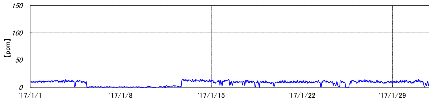
烧却炉 排ガスCO濃度[2017年1月実績]
