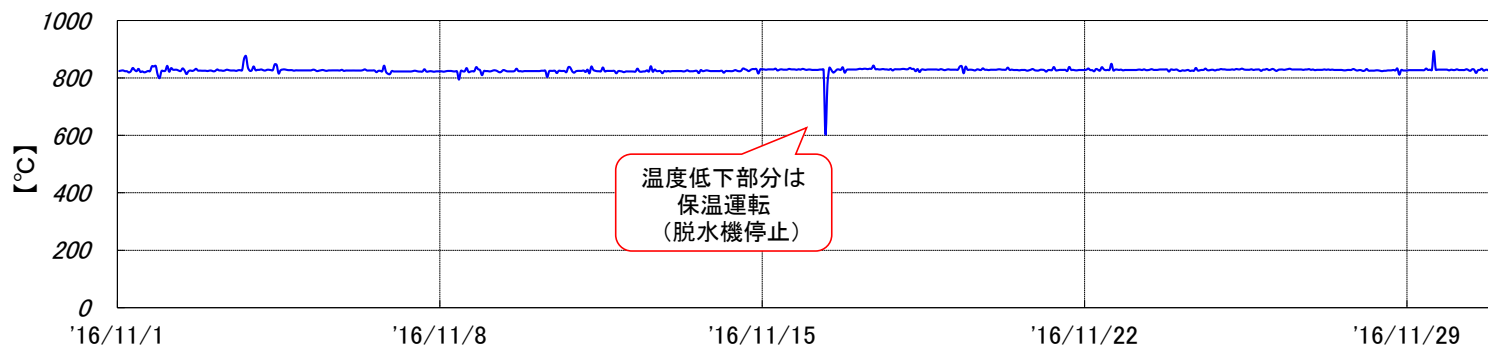
焼却炉 燃烧温度[2016年11月実績]
