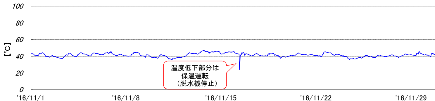
焼却炉 排ガス温度[2016年11月実績]
