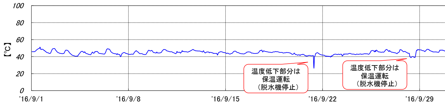
烧却炉 排ガス温度[2016年9月実績]
