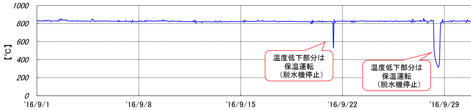
烧却炉 燃烧温度[2016年9月実績]
