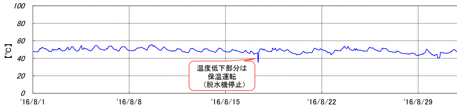
焼却炉 排ガス温度[2016年8月実績]
