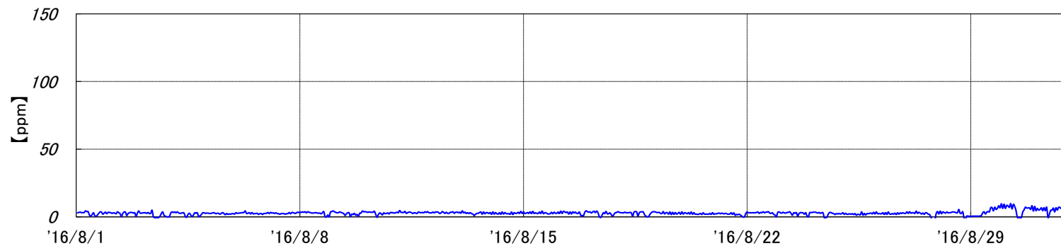
焼却炉 排ガスCO濃度[2016年8月実績]
