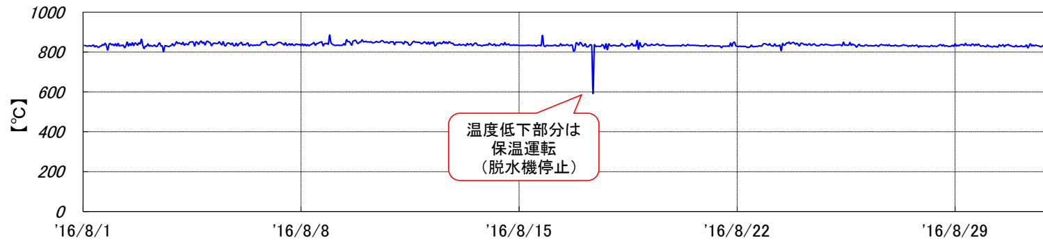
焼却炉 燃烧温度[2016年8月実績]
