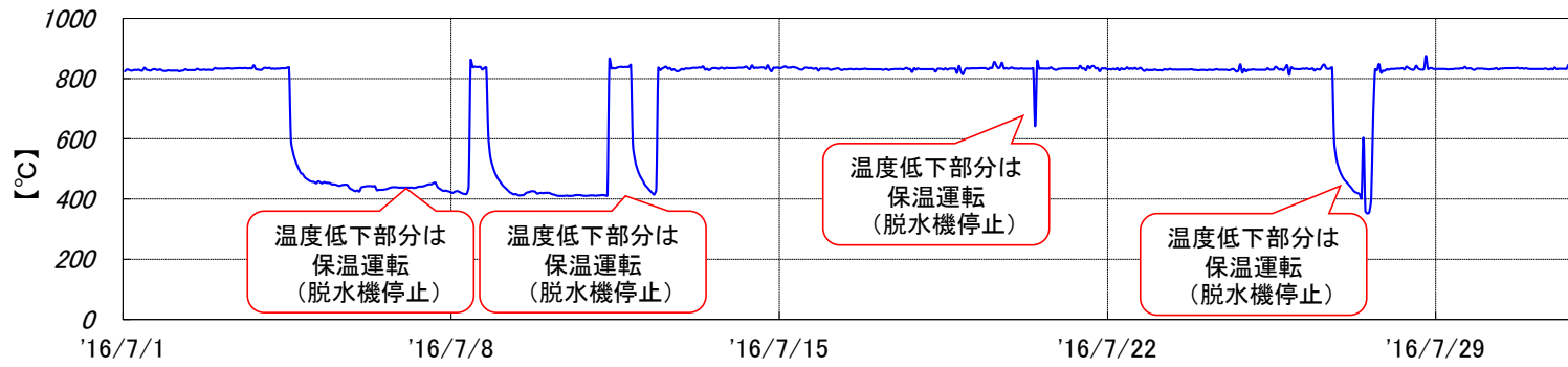
烧却炉 燃烧温度[2016年7月実績]
