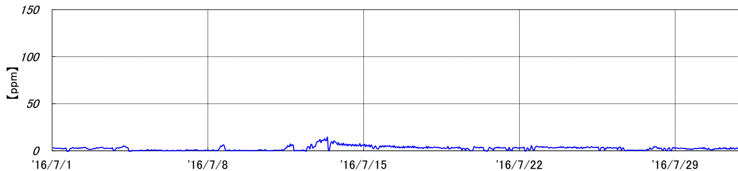
烧却炉 排ガスCO濃度[2016年7月実績]
