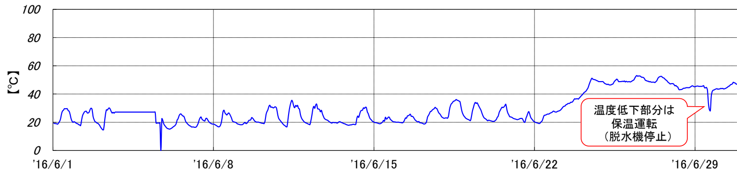
焼却炉 排ガス温度[2016年6月実績]
