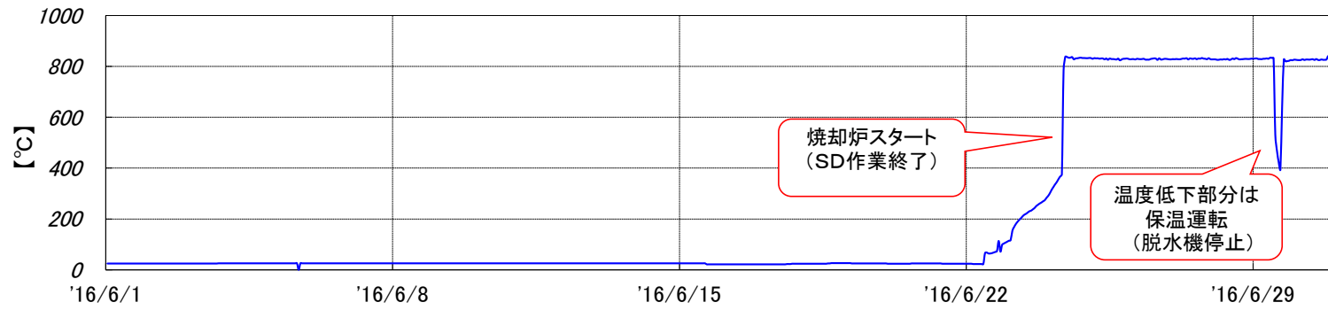
焼却炉 燃烧温度[2016年6月実績]
