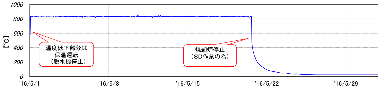
焼却炉 燃烧温度[2016年5月実績]
