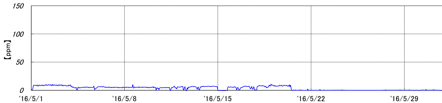
焼却炉 排ガスCO濃度[2016年5月実績]
