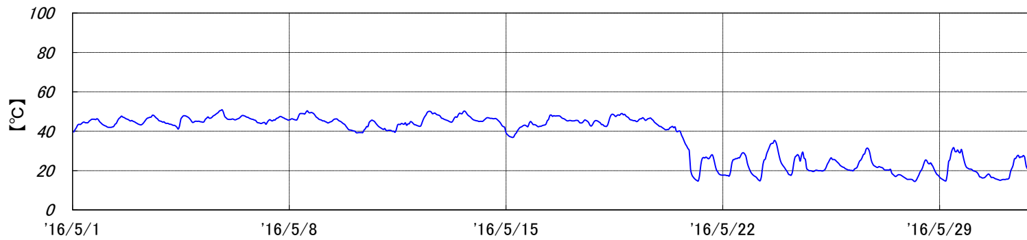
焼却炉 排ガス温度[2016年5月実績]
