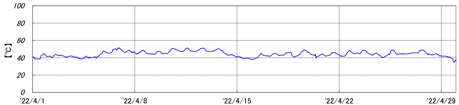
烧却炉 排ガス温度[2022年4月実績]
