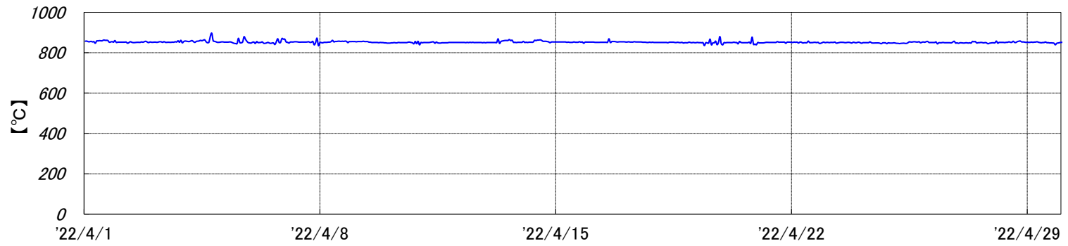
烧却炉 燃烧温度[2022年4月実績]
