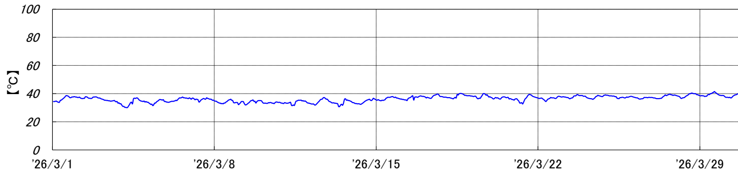
焼却炉 排ガス温度[2026年3月実績]
