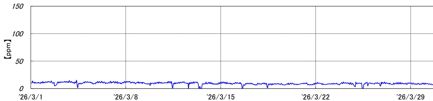
焼却炉 排ガスCO濃度[2026年3月実績]
